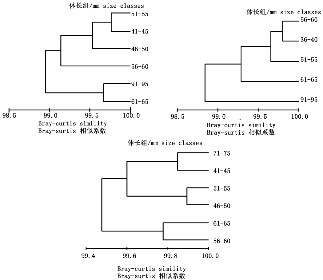
图 3 长江口及其邻近海域 3 个调查站 (A、C 和 E) 各个体长组虹鲮碳氮稳定同位素比值聚类分析图
