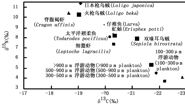
图 1 春季长江口海域虹鲮及其潜在饵料的 \delta^{13}C 和 \delta^{15}N 值
